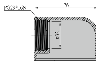
A-A 剖視圖
